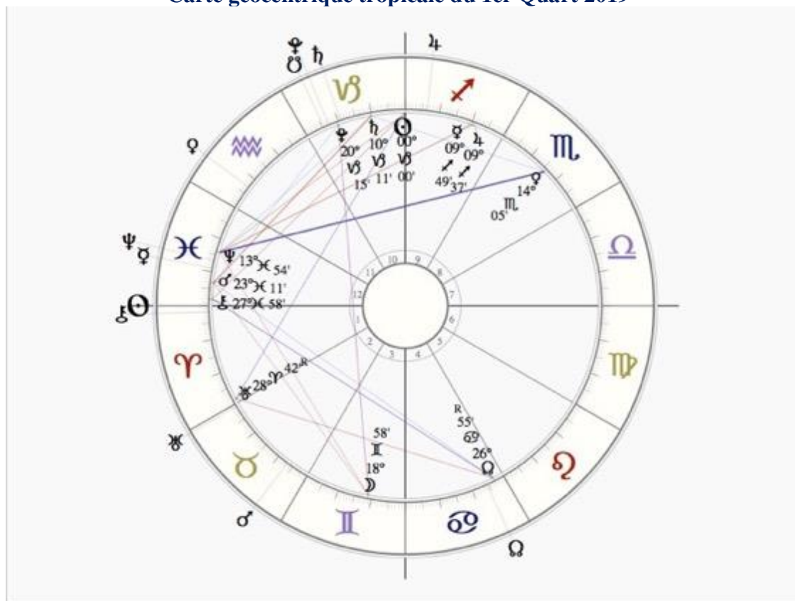
Roue interne : 21 déc. 2018 h. 22.23 UT – Roue externe : 20 mars 2019 h. 21.58
