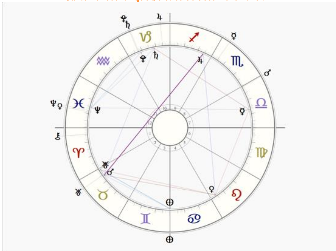
Roue interne : 21 déc. 2018 h. 22.23 UT – Roue externe : 22 déc. 2019 h 4.21
